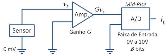
Figura 2. Esquemático do sistema de aquisição do exercício 2.
