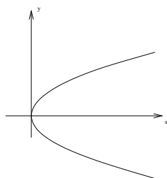
FIGURA 11. Conjunto \{(x, y) \in \mathbb{R}^2 : x = y^2\} .
